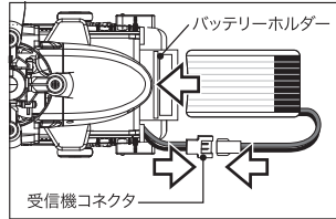
②機体側の受信機コネクタとバッテリーのコネクタを、極性に注意して接続し、バッテリーをバッテリーホルダーに収納します。
