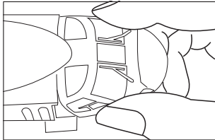
①ヘッドカバーを外します。
